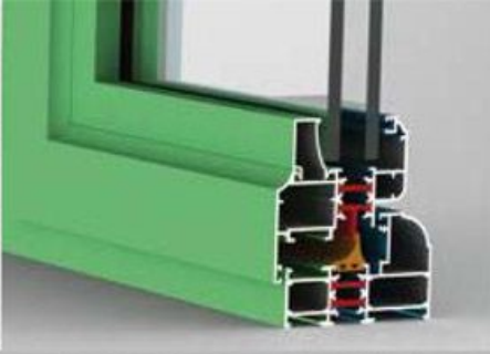
دیتیل یراق آلات پنجره لولایی ترمال بریک سری TH 75L Thermal break hinged window fittings of series TH 75L (detail)
